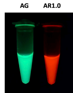
図3 改変前と改変後の蛍光蛋白質
