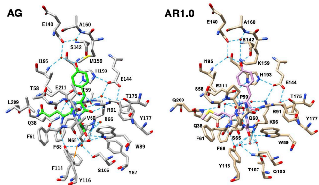
図4 発色団周辺の構造
